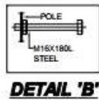
POLE 연결 상세도
