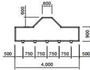
A-A DETAIL
