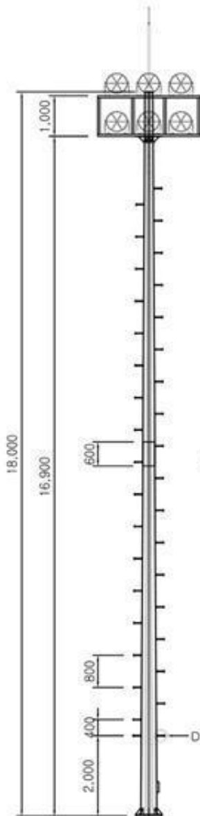
POLE 연결 상세도
