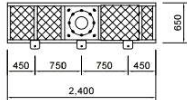
B- 'B' DETAIL
